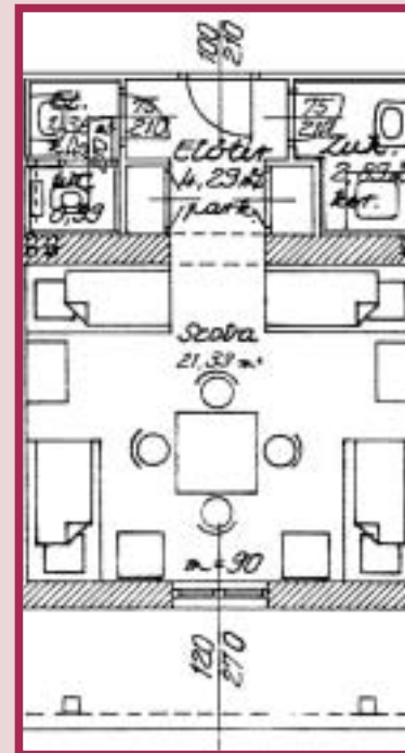
Egy 8 ágyas szoba alaprajza
